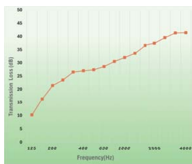
STC:31 隔音性能圖
