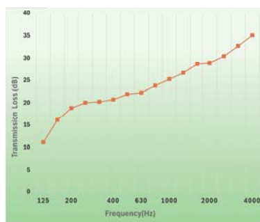
STC:26 隔音性能圖
