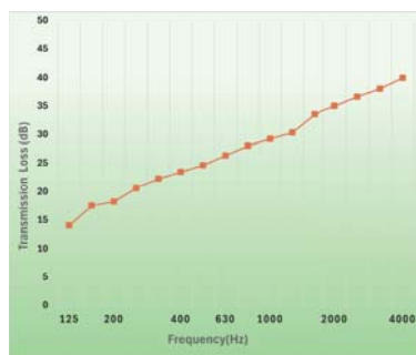
STC:29 隔音性能圖
