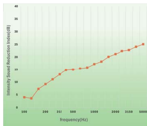
Rw=18 隔音性能圖
