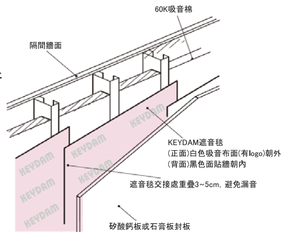
遮音毯施工簡易圖
