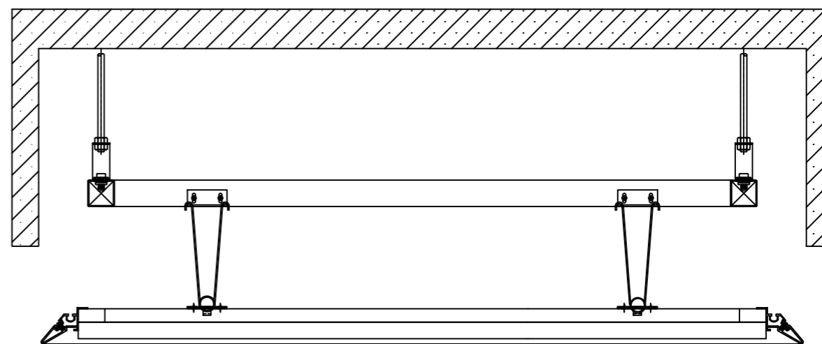
維護拆卸示意圖
