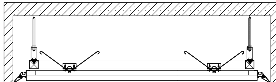
安裝完成示意圖
